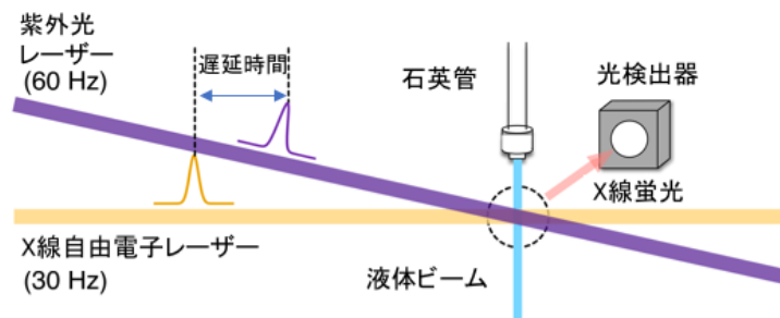
図 1 時間分解 X 線吸収スペクトル測定装置概略図
