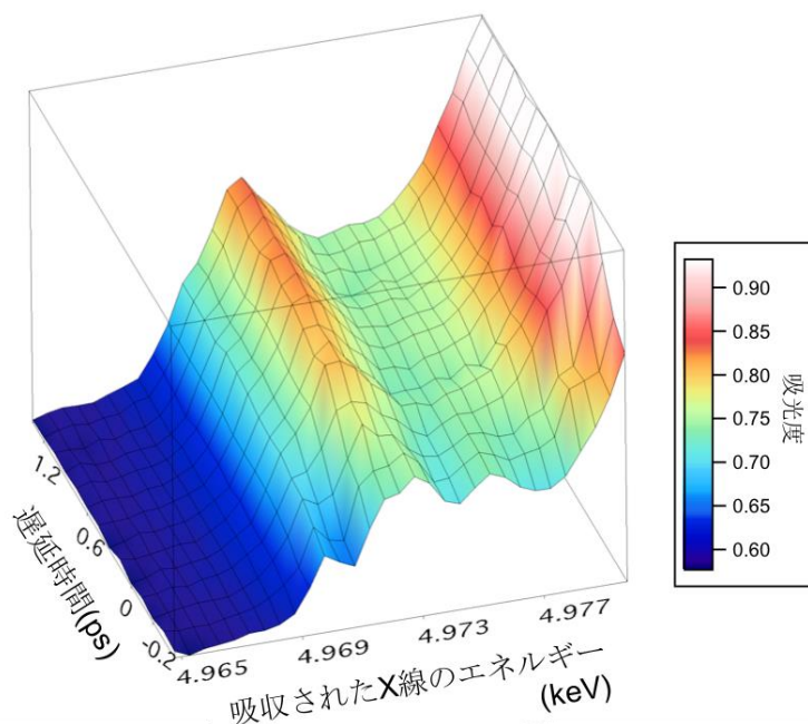
図 2 X線吸収スペクトルの時間変化
